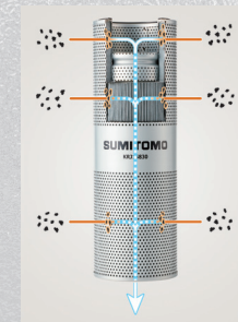
リターンフィルタの詳細
