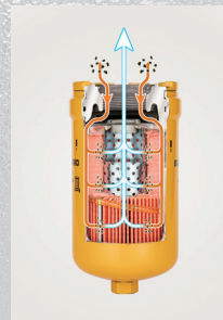
パイロットラインフィルタの詳細
