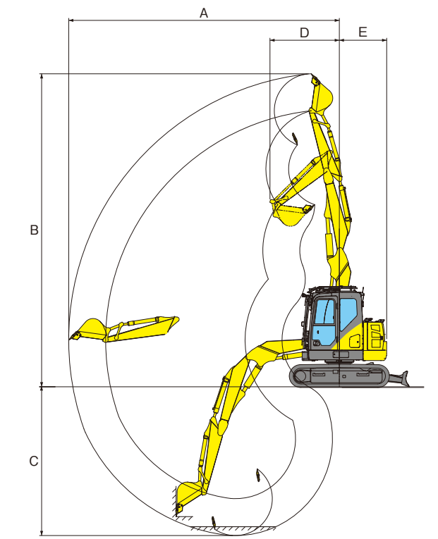
SH75X-7KK作業範囲図(バケット)
