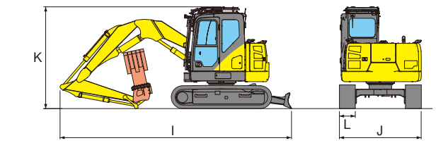
SH75X-7KK外形寸法図(フォーク)
