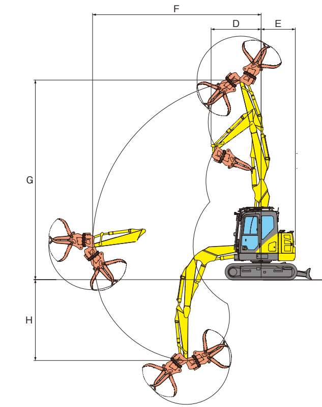
SH75X-7KK外形寸法図(フォーク)
