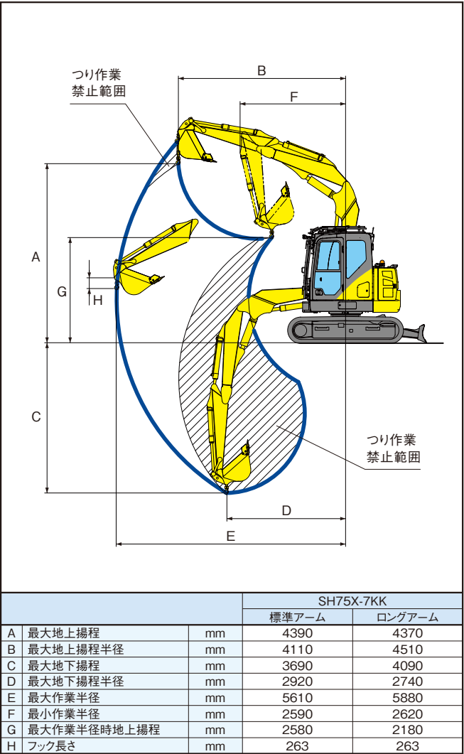
クレーン仕様作業範囲図
