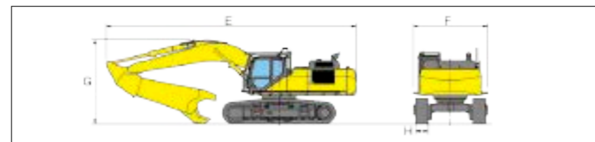
■外形寸法図 SH480LHD-6
