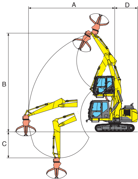
■作業範囲図
