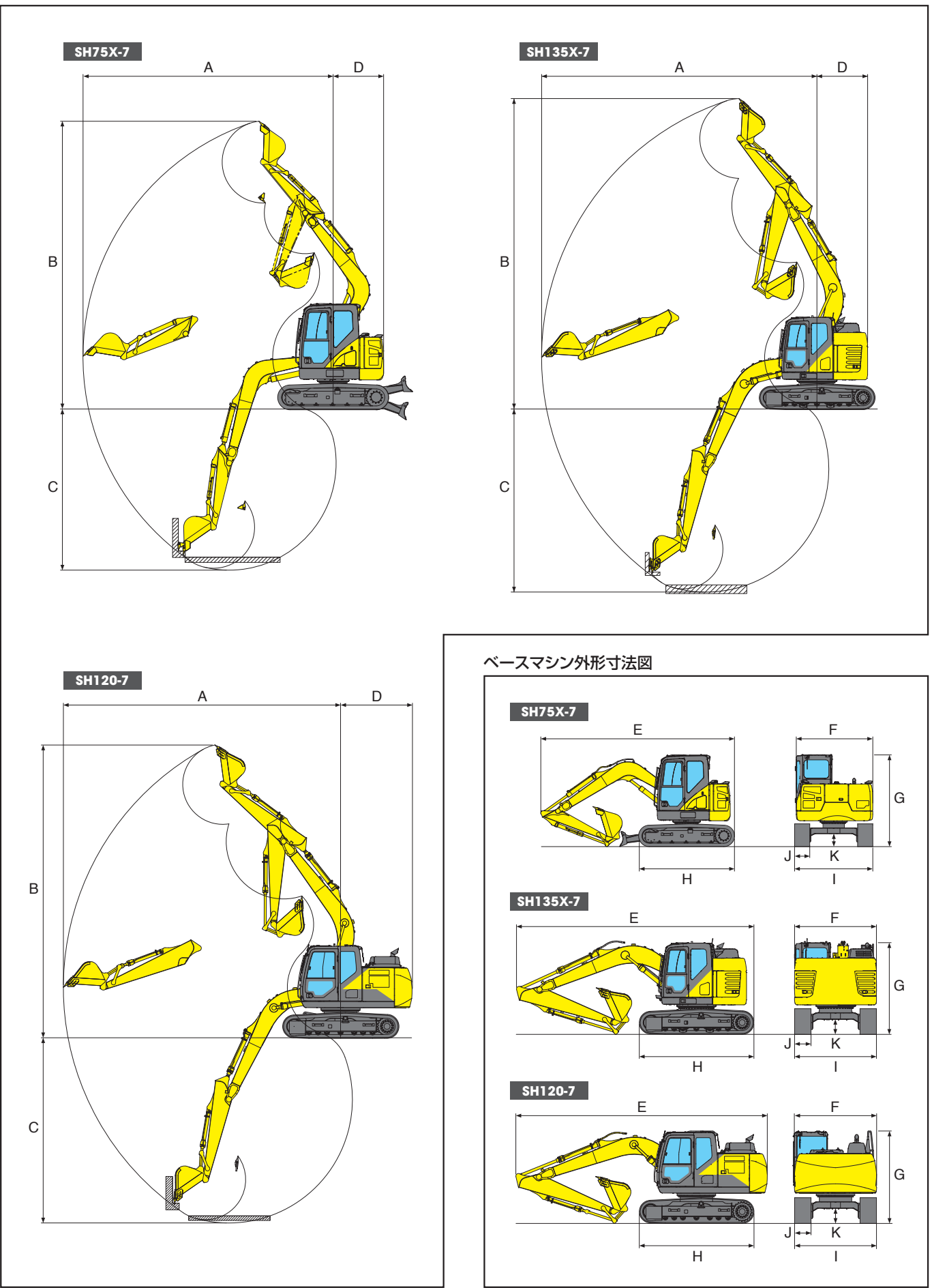
ベースマシン作業範囲図
