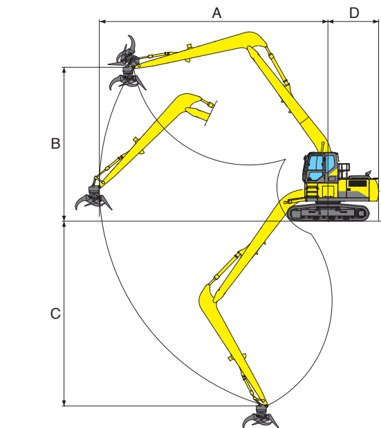
■作業範囲図
