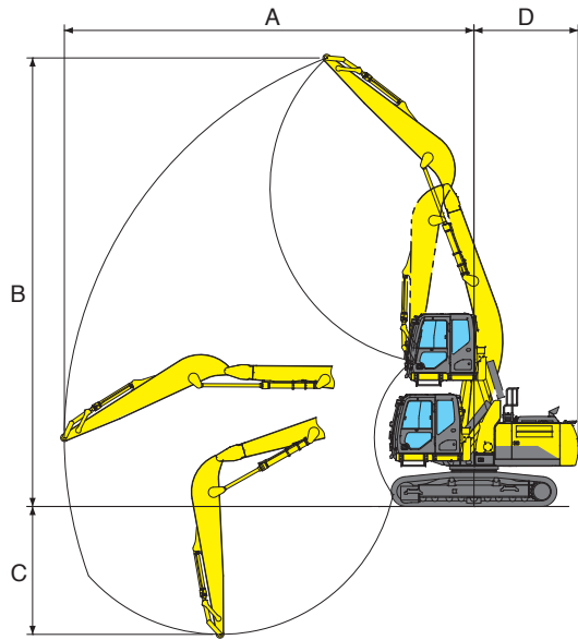
■作業範囲図
