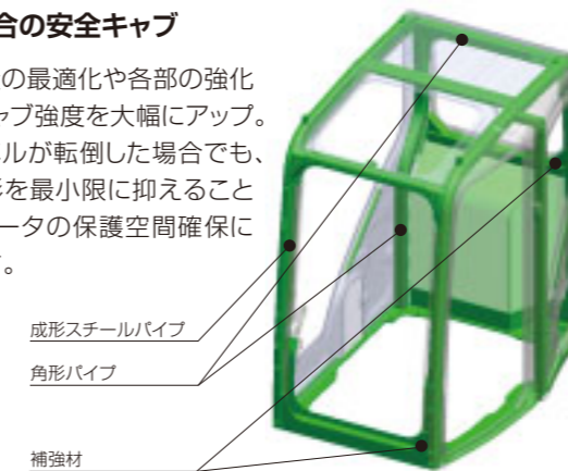
補強材
