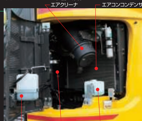
エアクリーナ エアコンコンデンサ リザーブタンク リレーボックス ウォッシュタンク
