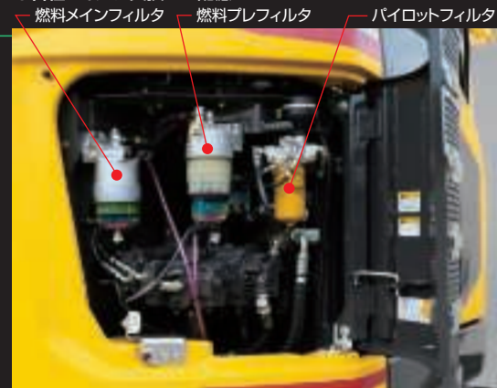
燃料メインフィルタ 燃料プレフィルタ パイロットフィルタ
