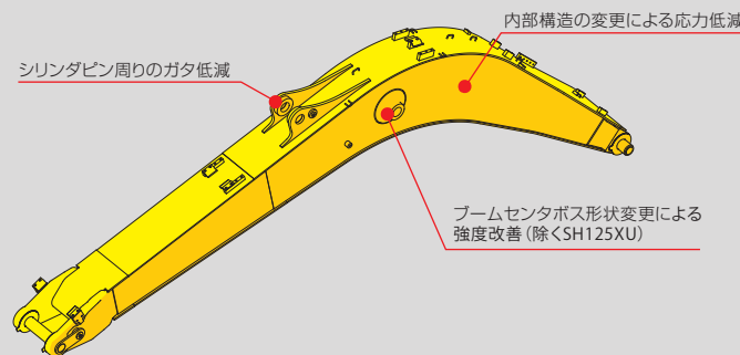
内部構造の変更による応力低減
